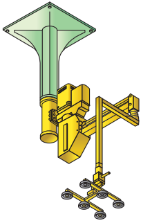
天井固定式
