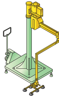
パレトラ式
